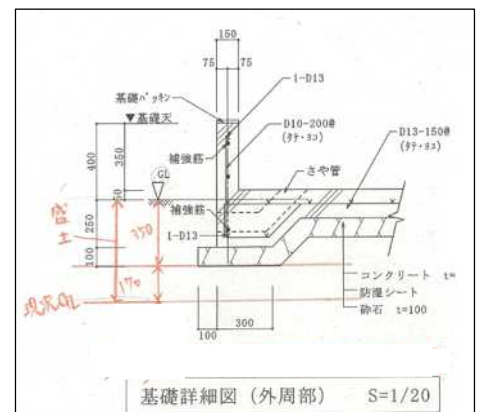
断面図記入例
