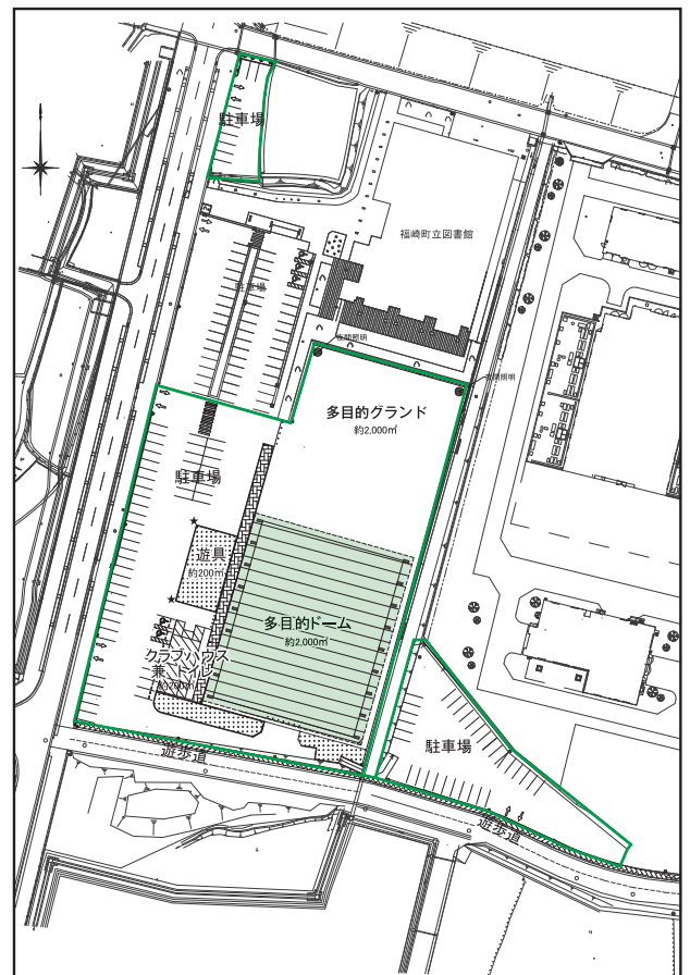
多目的グランド配置図(案)
