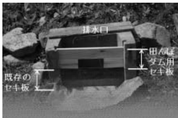
せき板設置状況
