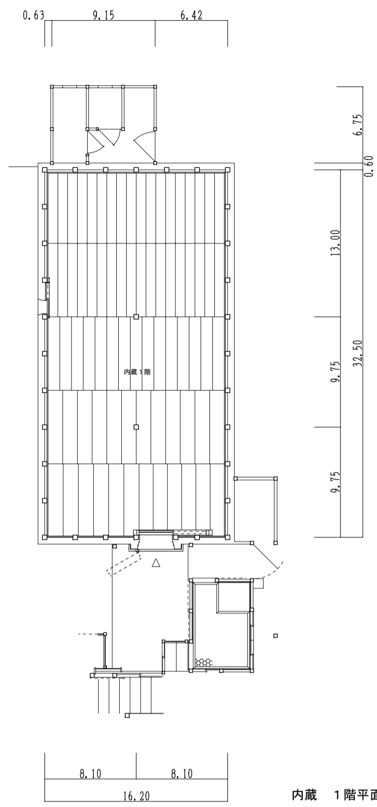
内蔵 1階平面図
