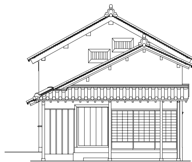
酒造蔵 南立面図
