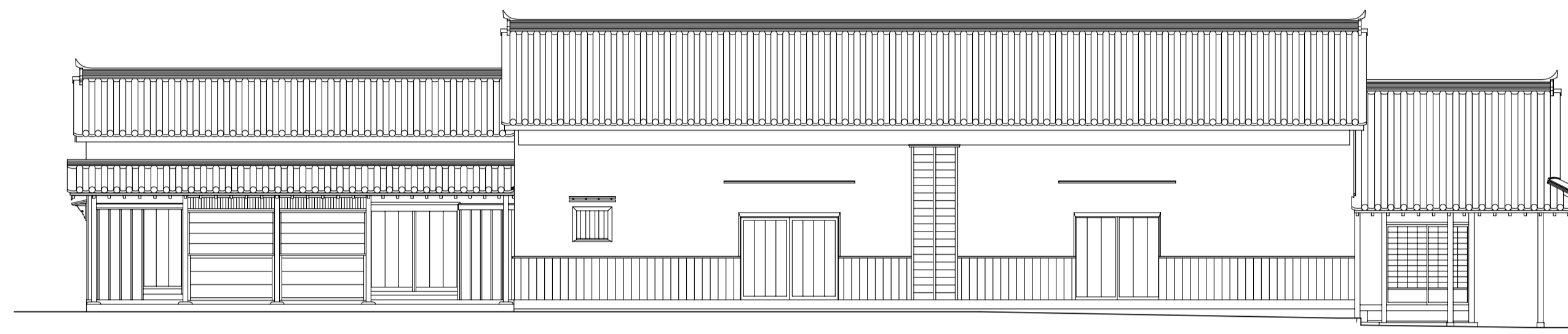
酒造蔵 西立面図
