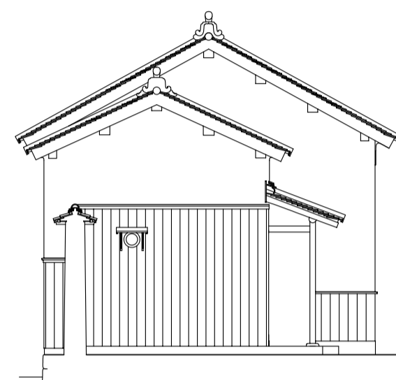
酒造蔵 北立面図
